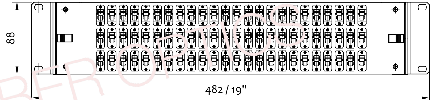
72x E2000 (FRONT VIEW)
